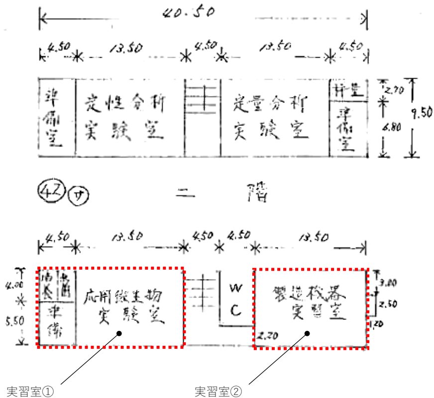
[食品デザイン科教棟平面図]
